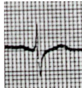
aVR
