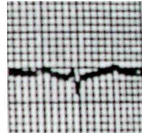
aVF
