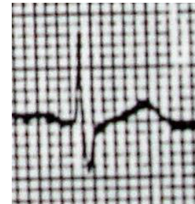
aVL
