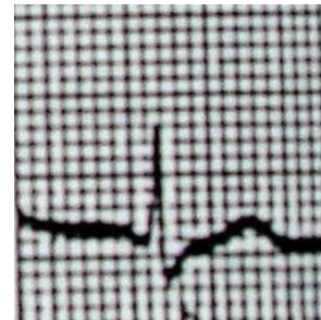
aVF
