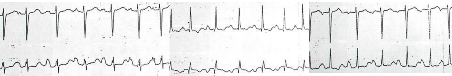
aVL & aVF
