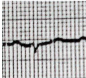
DIII
