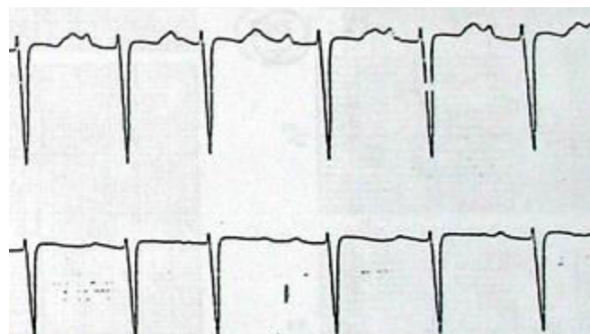
V3& V4
