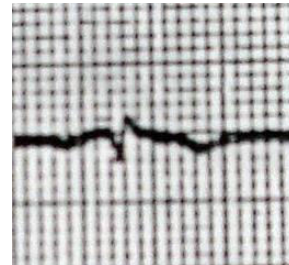
aVR
