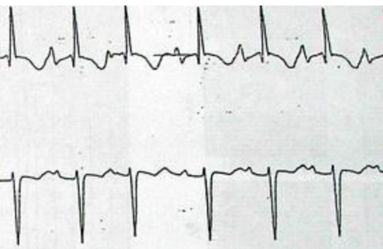
V1 & V2
