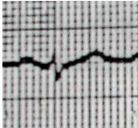
DII
