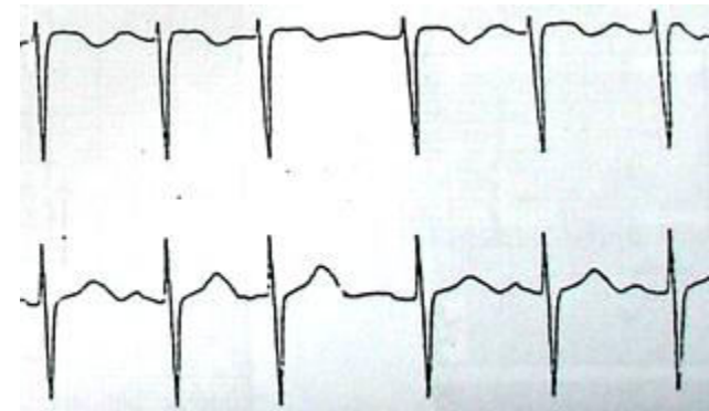
V5& V6
