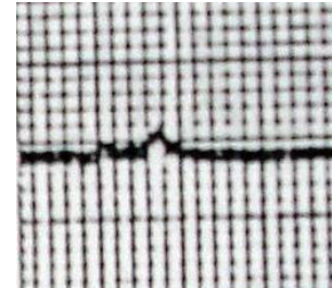
aVL
